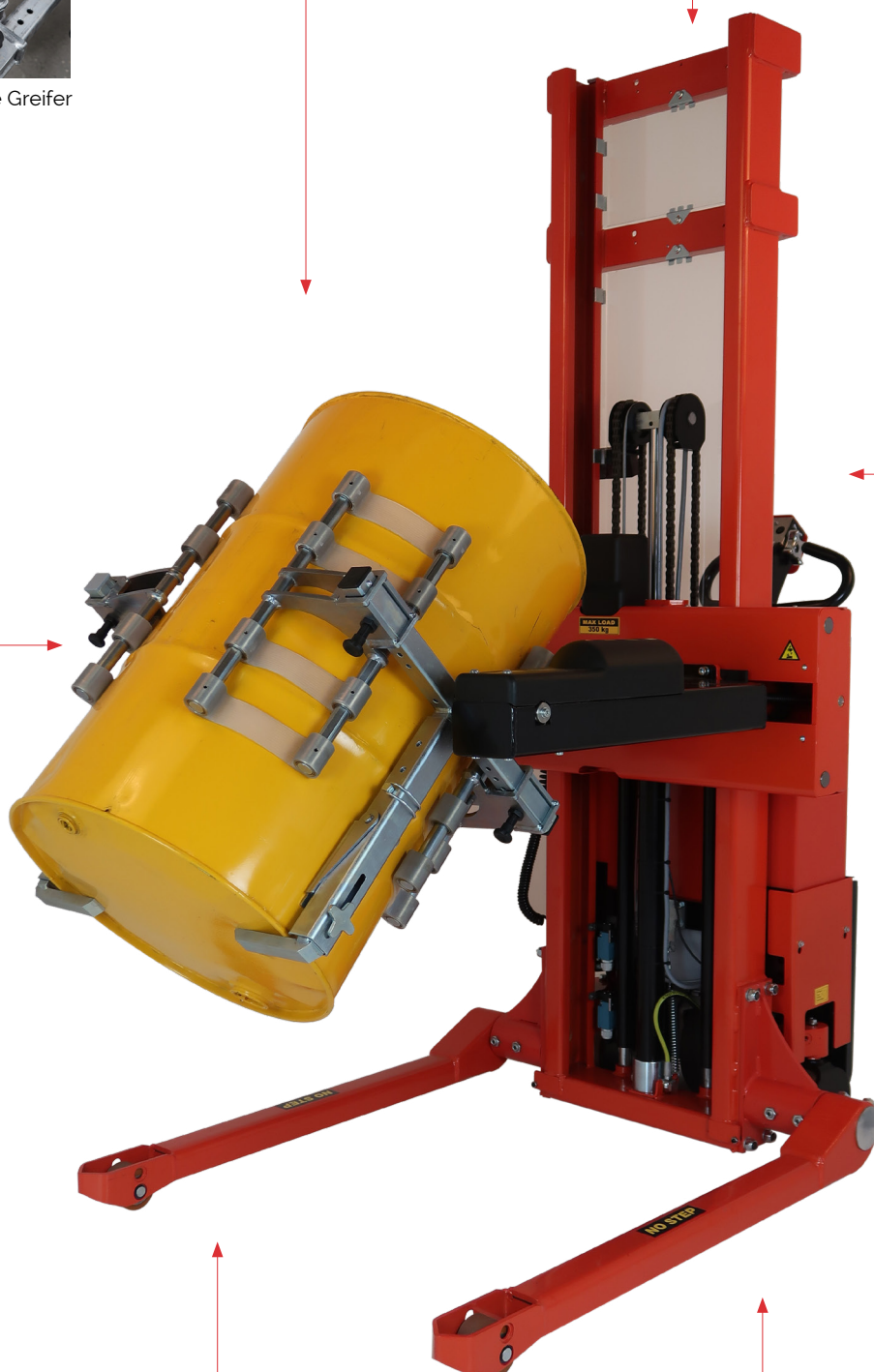
Fernbedienung für elektrisches Festspannen, Heben, Senken und Rotation
