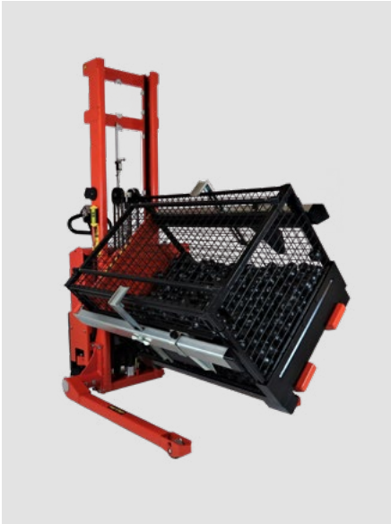
Rotator mit einstellbaren Boxhaltern
